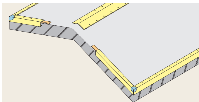
1. DN 鋼板の取付け
