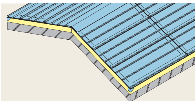
6. 端部処理(シーリング材)
