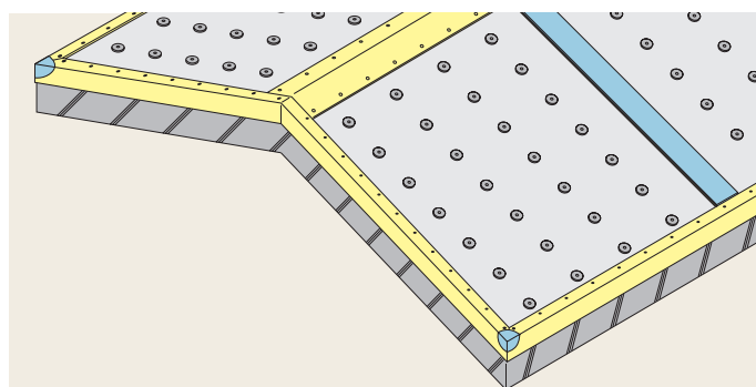
3. DN 鋼板へのベルトシート溶着
