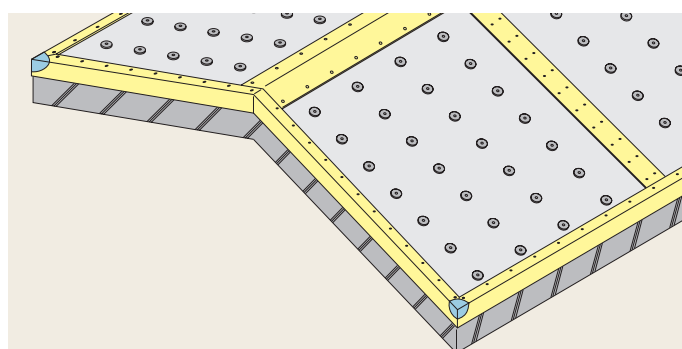
2. ディスク板・DN 鋼板の取付け
