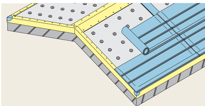
4. ダンスラントルーフ敷込み
